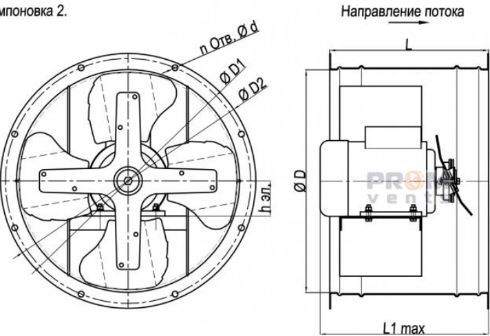
Компоновка 2.
