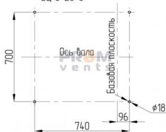
Схема расположения отверстий для крепления вентилятора ВЦ 6-20-8
